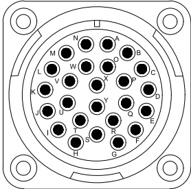
输出连接器
