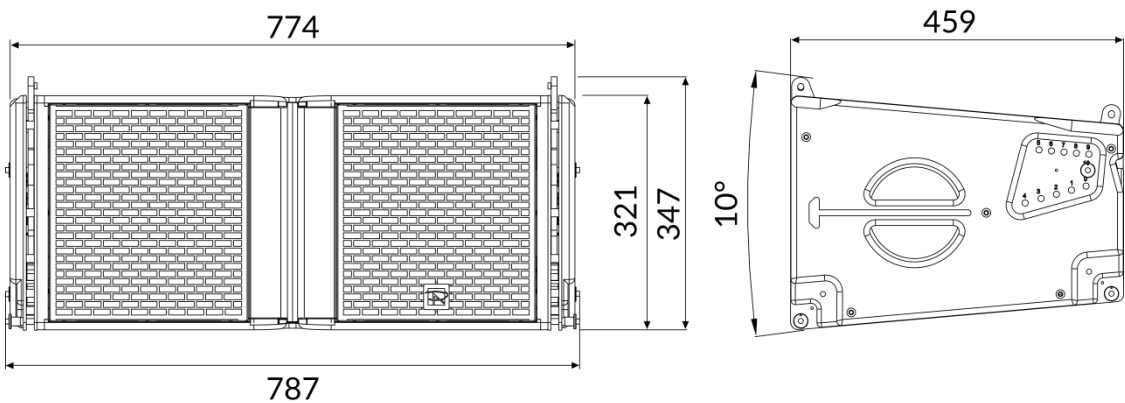
尺寸图 (mm)
