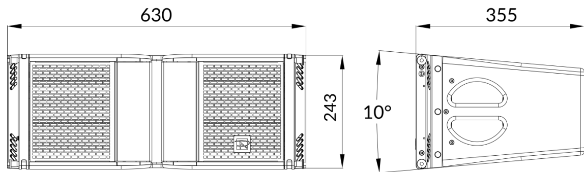
尺寸图 (mm)
